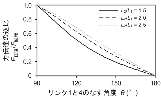
図4 力伝達の逆比 ( F_{\text{往復}}/F_{\text{回転}} )
