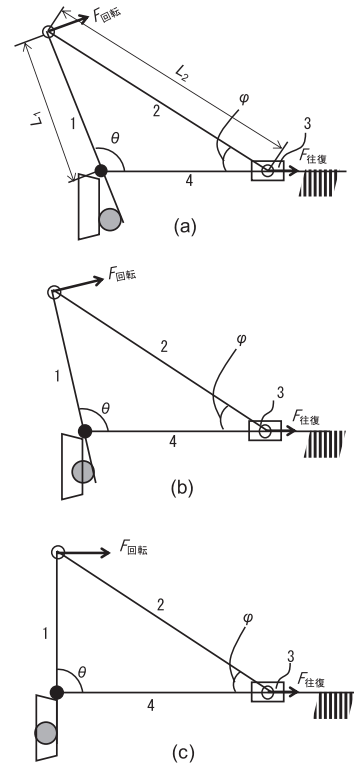
図3 引くことで動作する農業ハサミ構造 数字はリンクの番号である。灰色丸は作物茎を示す。黒丸、白丸のそれぞれは固定ピン、可動ピンを示す。パネルは切断の (a) 前、(b) 途中、(c) 後である。
